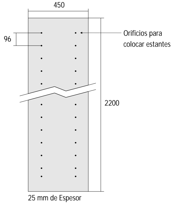
6305 Panel con cremallera simple empotrada (p/ utilizar con accesorios a cremallera)
