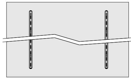
6305 Panel con cremallera simple empotrada (p/ utilizar con accesorios a cremallera)
