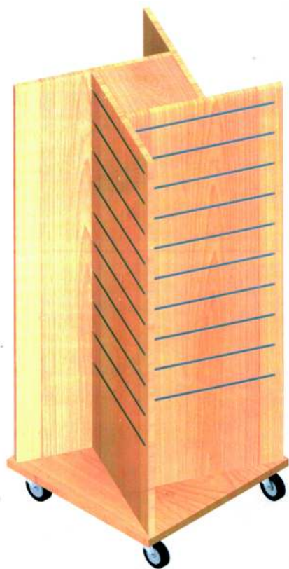
6708 Góndola c/ ruedas a cuatro caras. (1) Dim 540 x 540 x 1370 (h)
