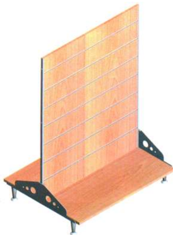
6711 Góndola c/ patas a dos caras. (1) Dim 930 x 740 x 1343 (h)
