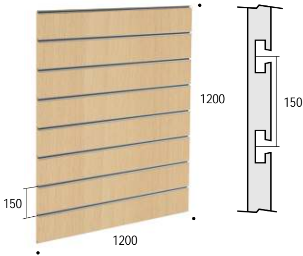
6701 Panel de lamas. Dim 1200 x 1200
