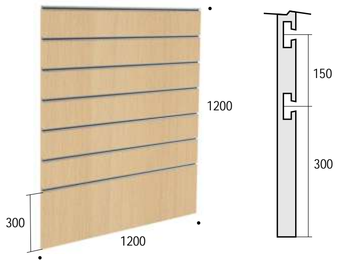
6702 Panel de lamas. Dim 1200 x 1200
